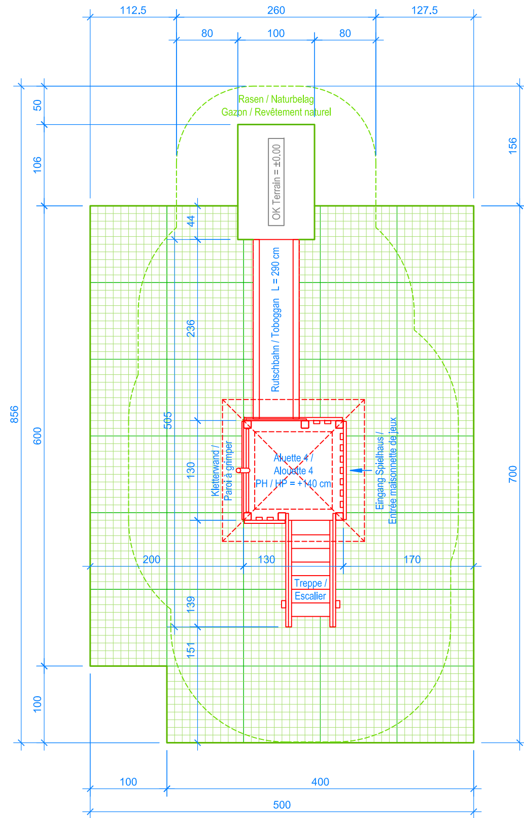
GRUNDRISS / PLAN 1:50
