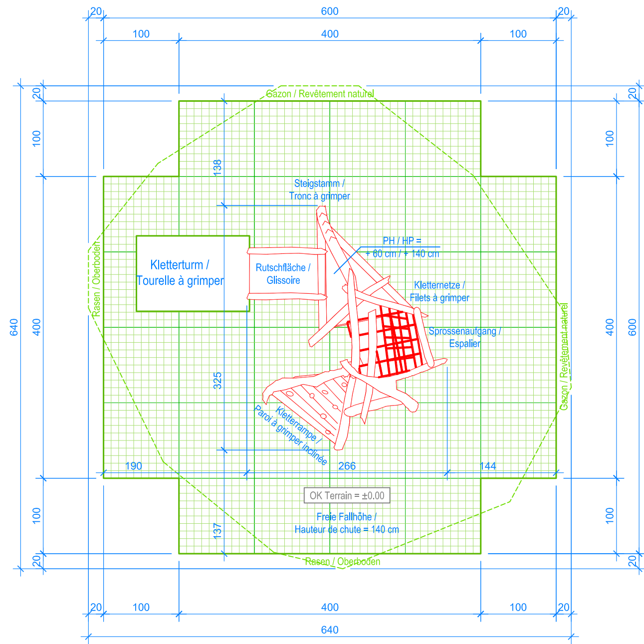
GRUNDRISS / PLAN 1:50
