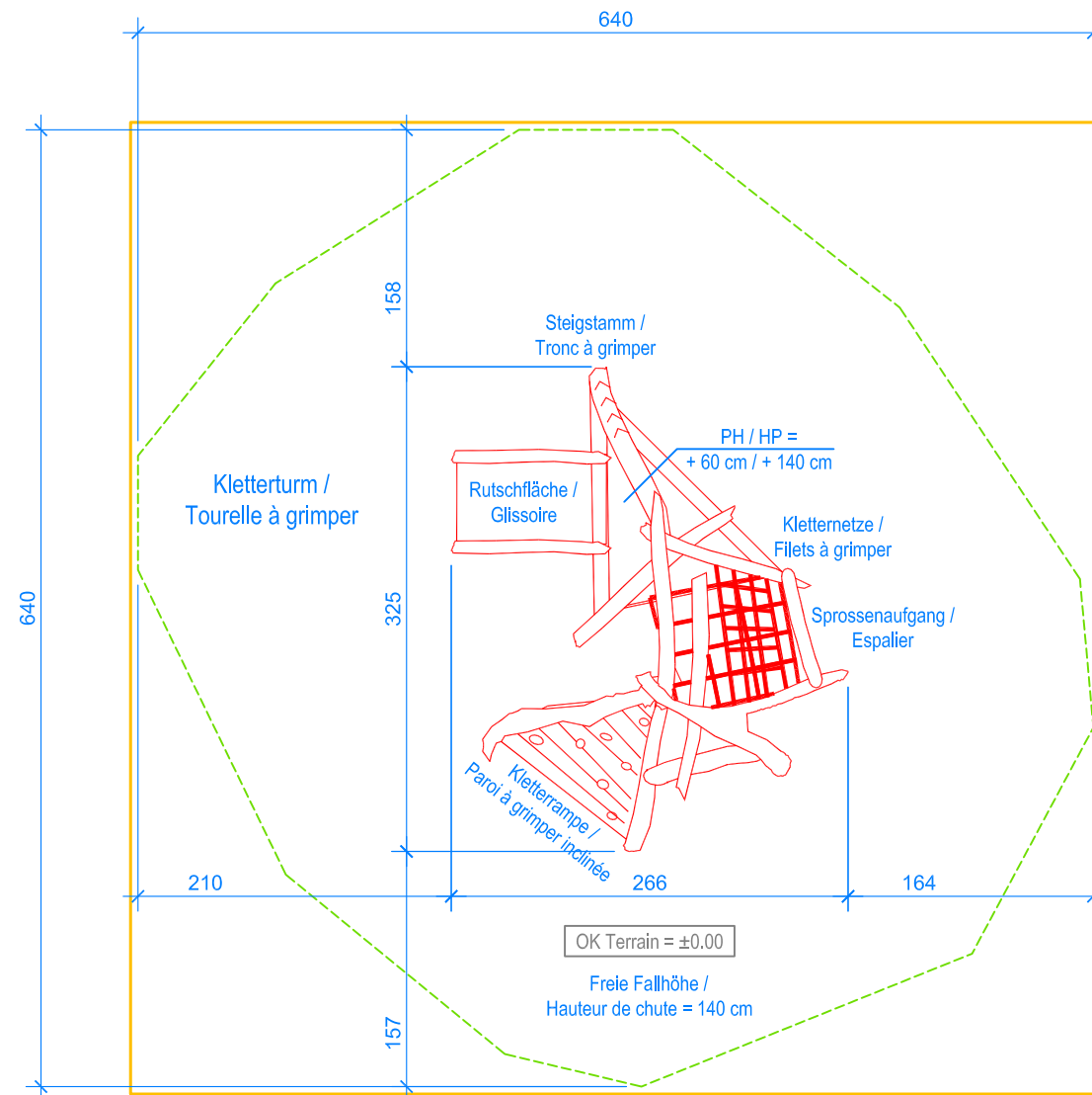
GRUNDRISS / PLAN 1:50
