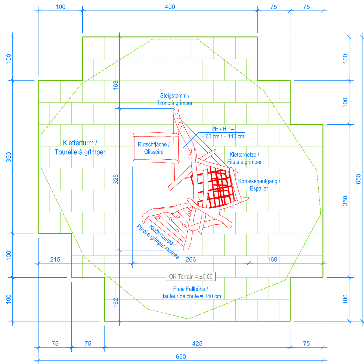
GRUNDRISS / PLAN 1:50
