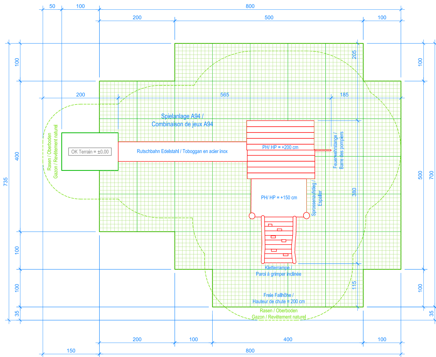
GRUNDRISS / PLAN 1:50
