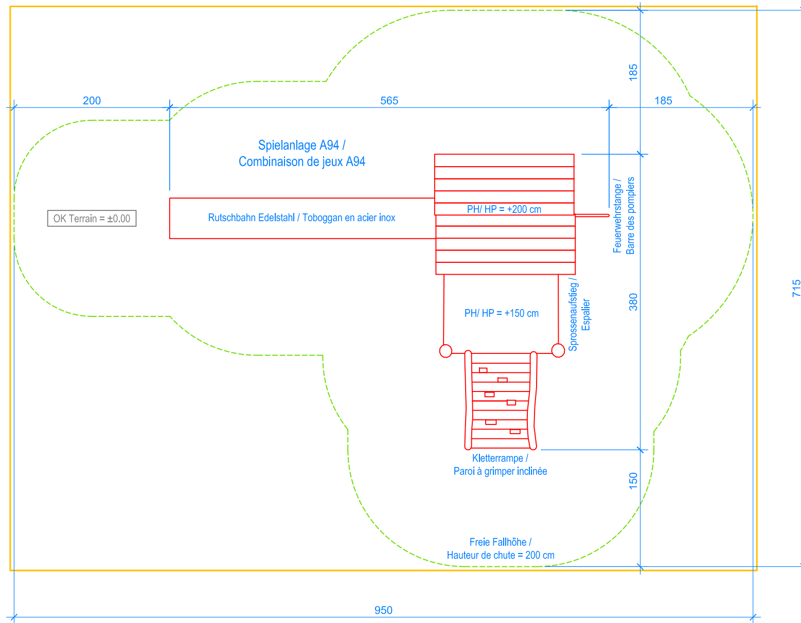
GRUNDRISS / PLAN 1:50
