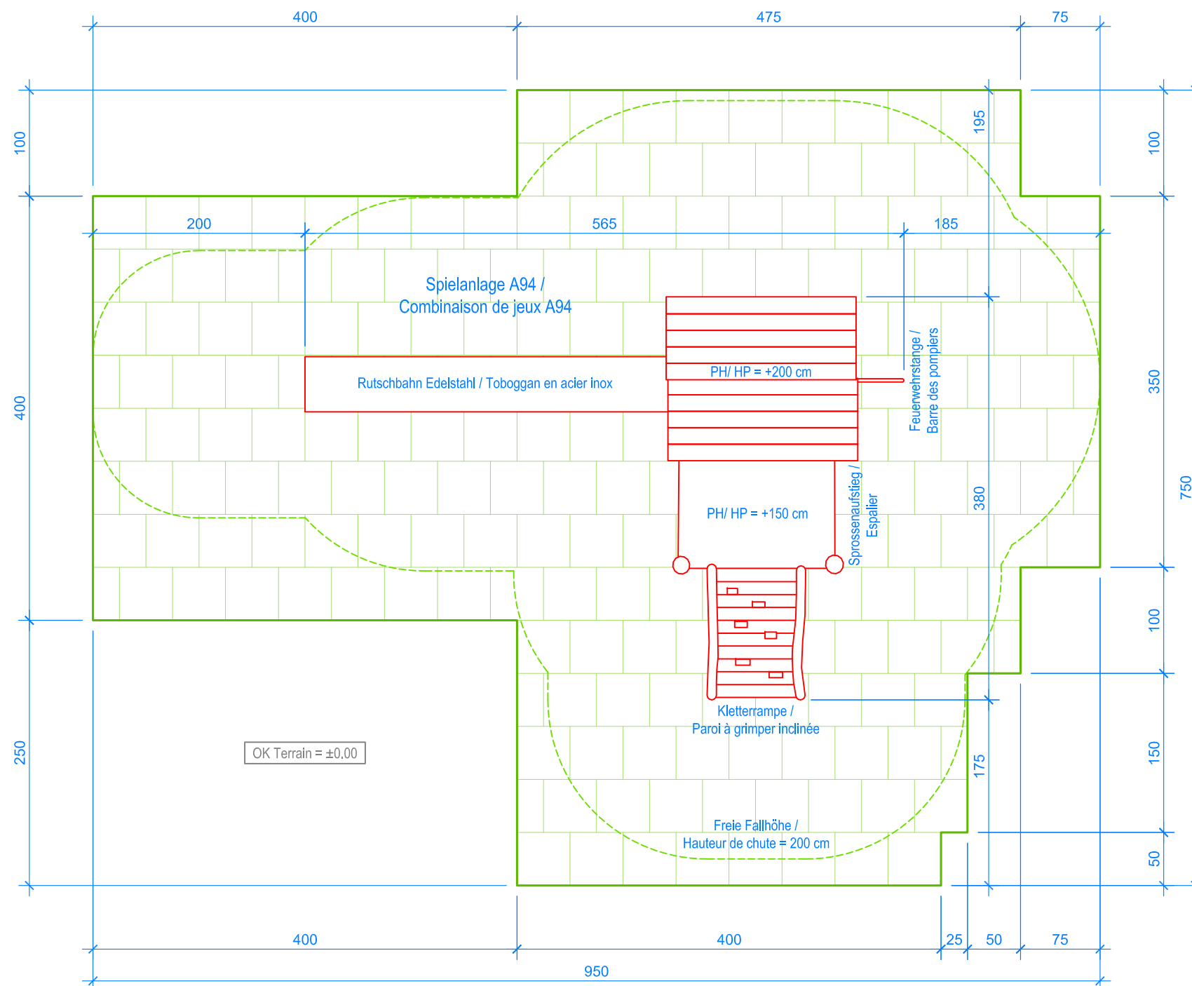
GRUNDRISS / PLAN 1:50
