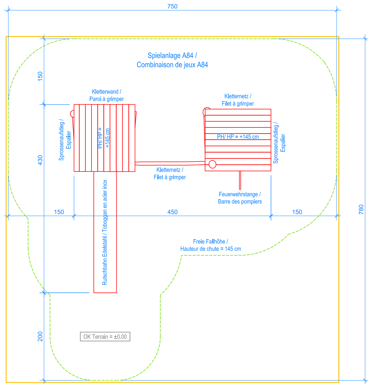
GRUNDRISS / PLAN 1:50
