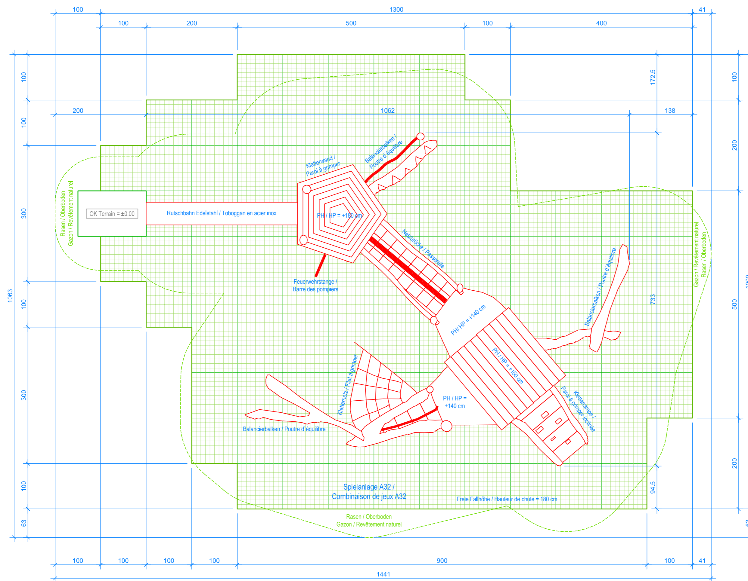
GRUNDRISS / PLAN 1:50
