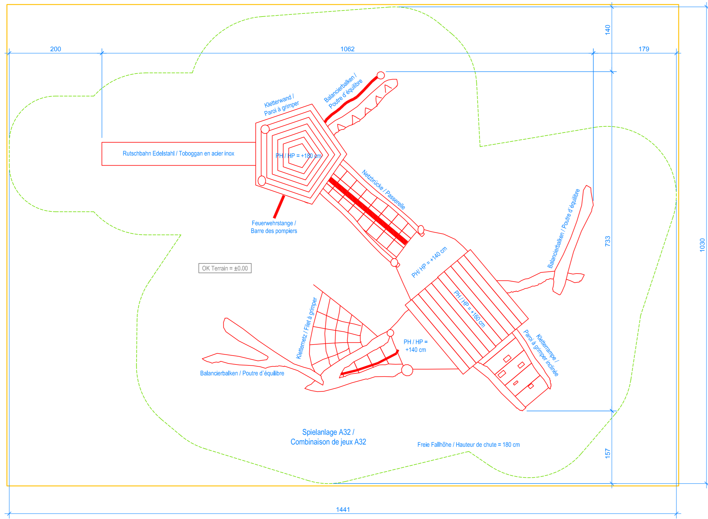
GRUNDRISS / PLAN 1:50
