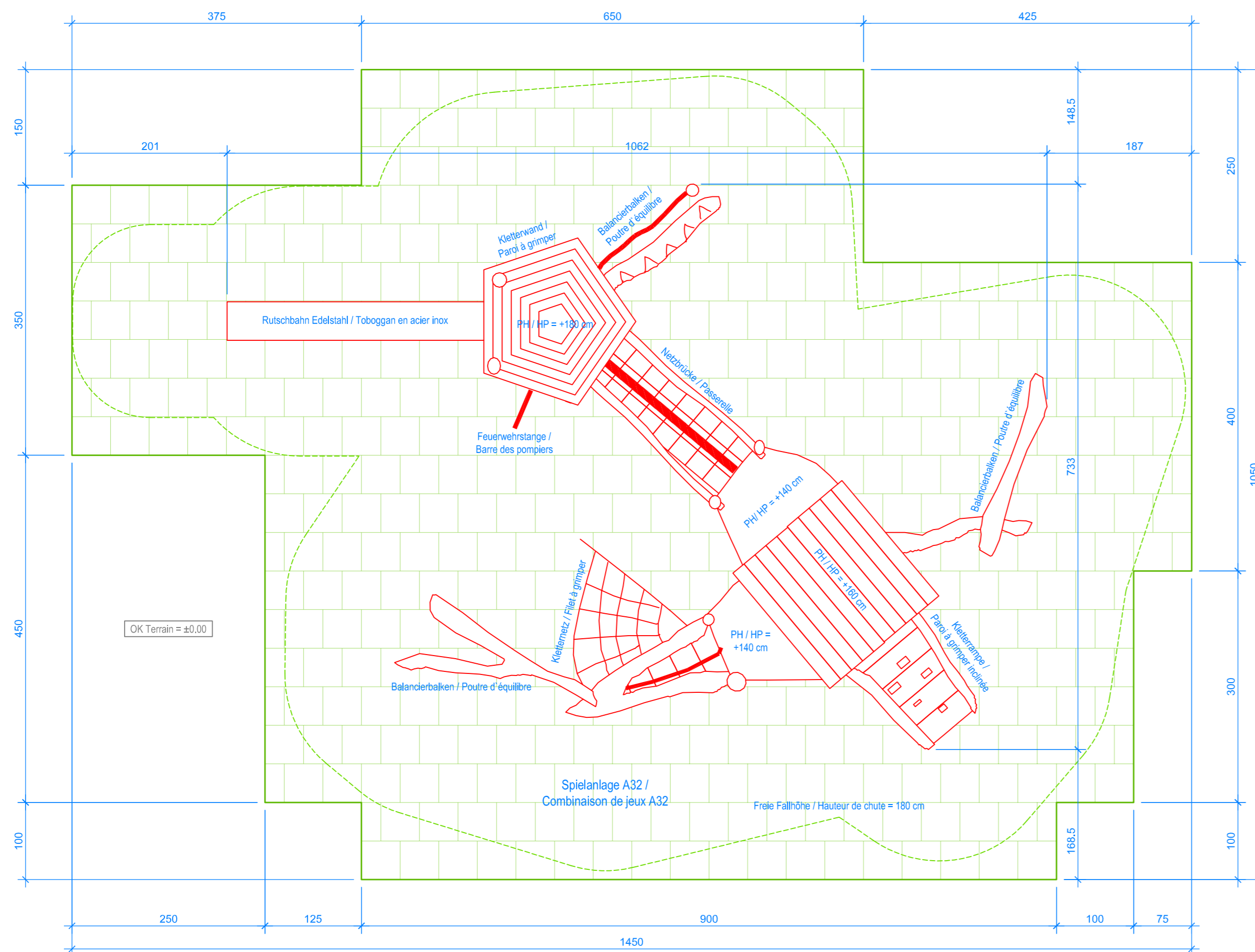
GRUNDRISS / PLAN 1:50
