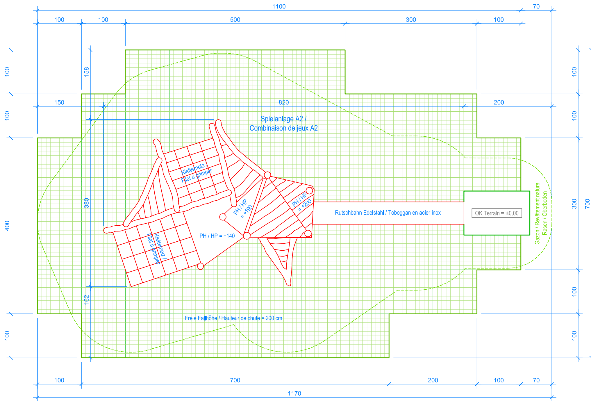
GRUNDRISS / PLAN 1:50
