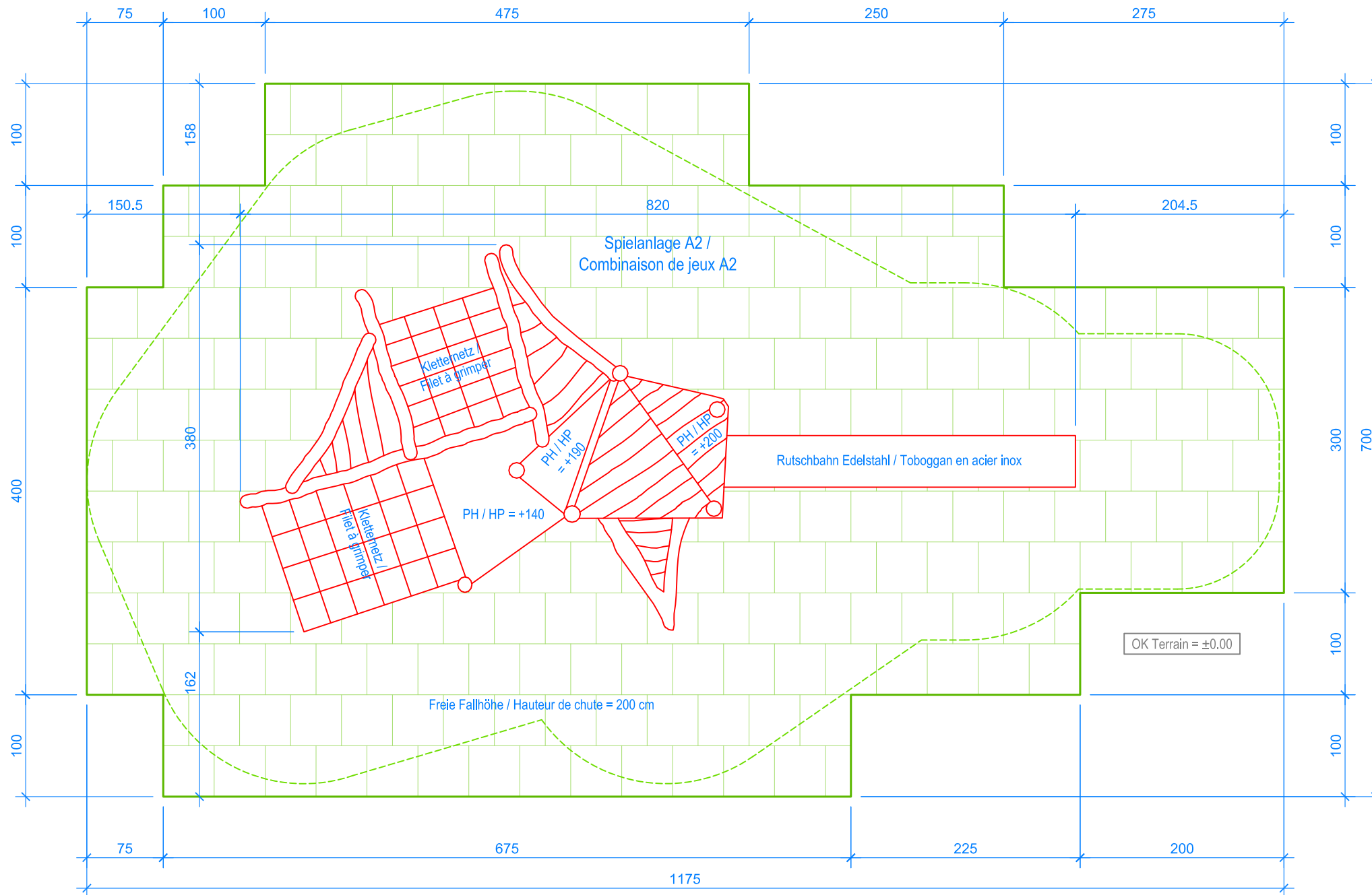
GRUNDRISS / PLAN 1:50
