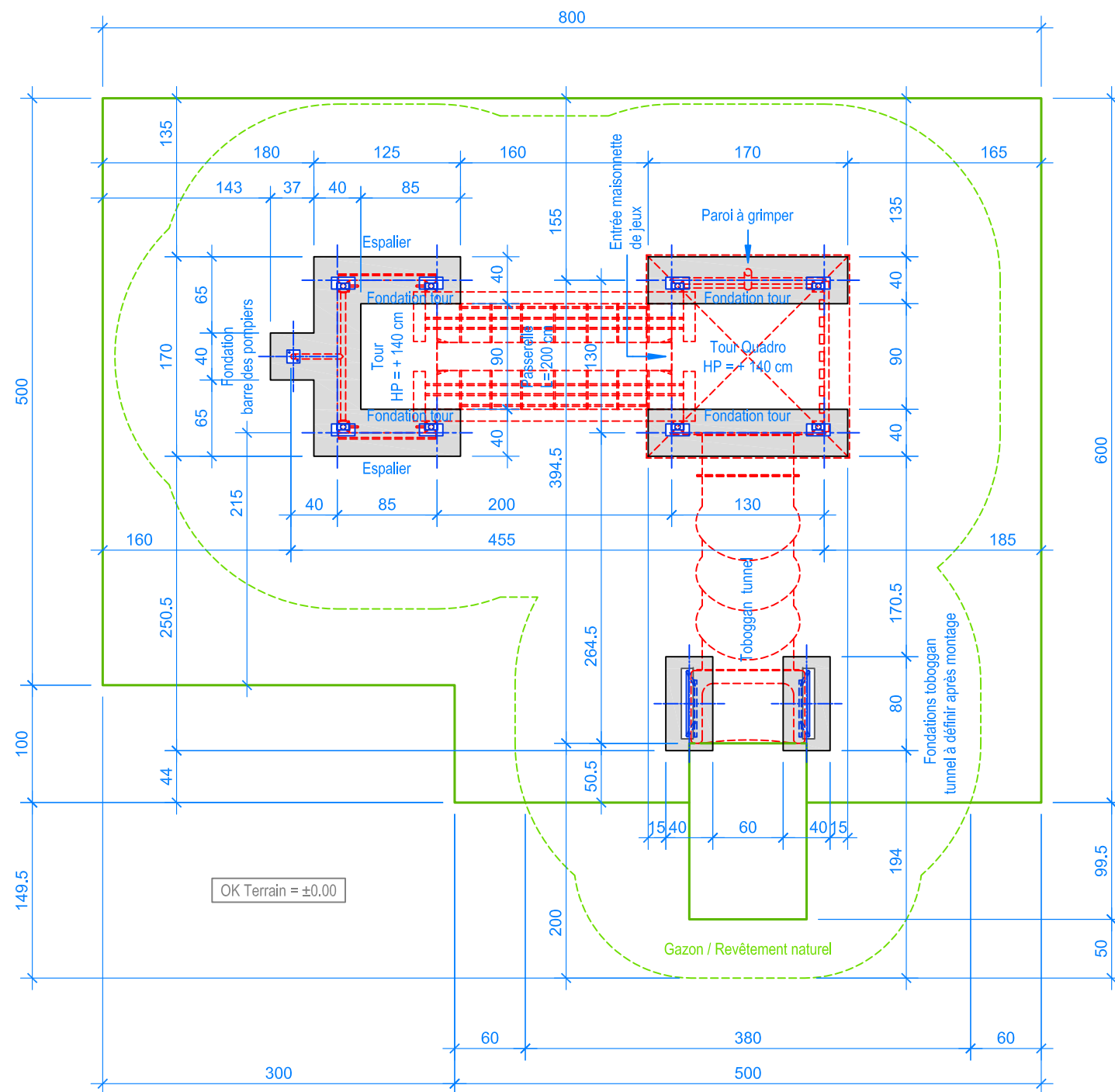
PLAN 1:50
