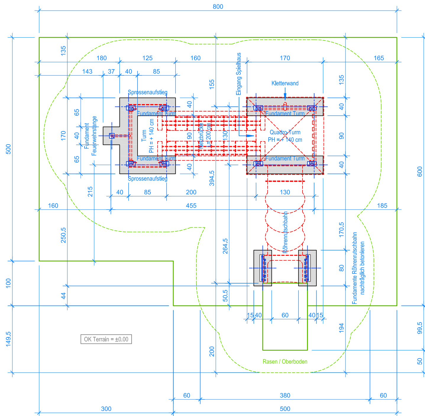
GRUNDRISS 1:50
