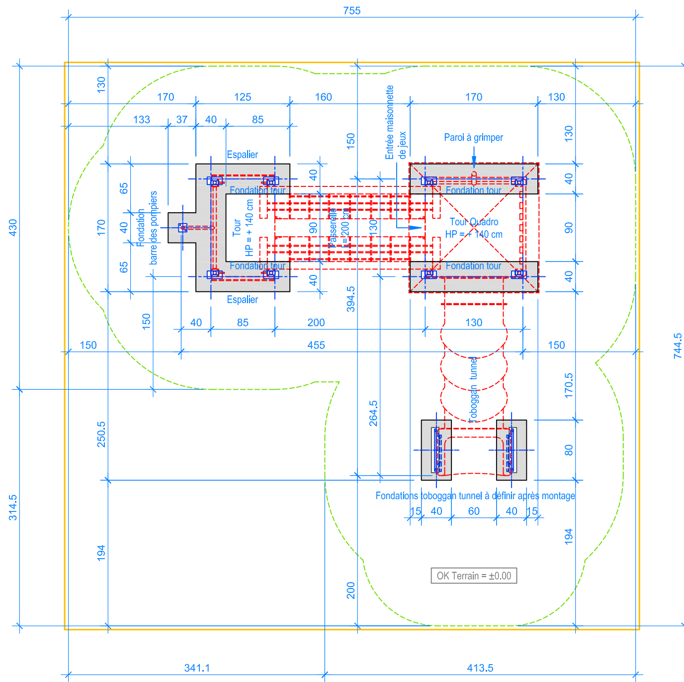
PLAN 1:50
