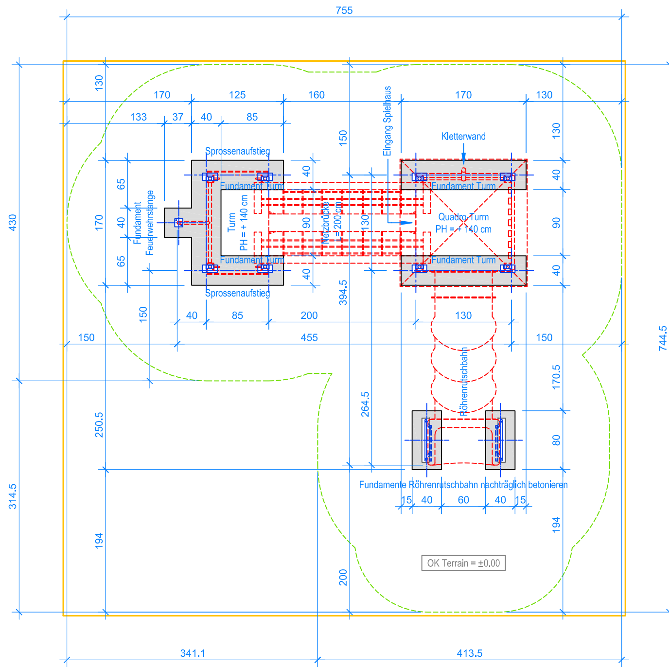
GRUNDRISS 1:50
