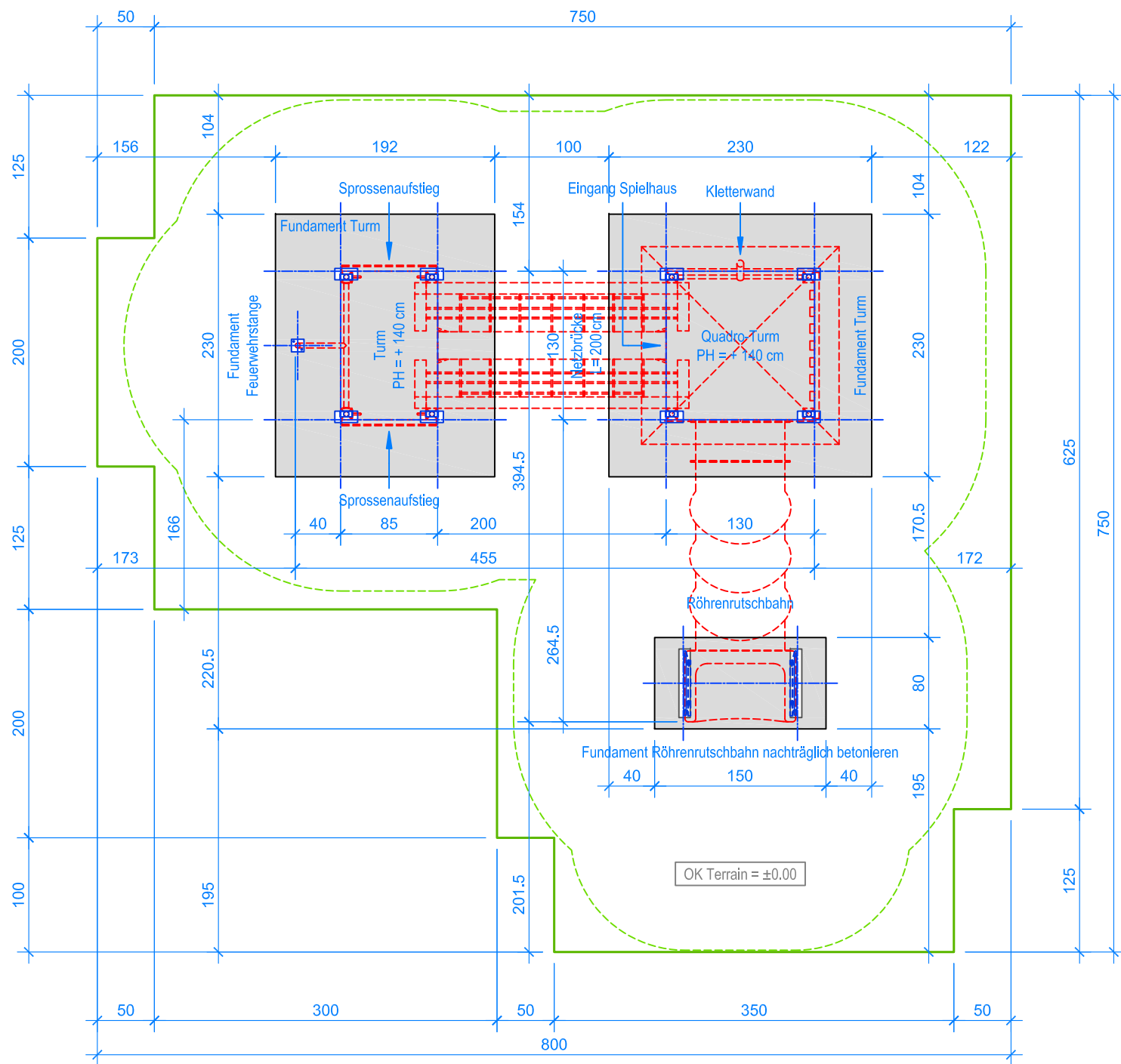
GRUNDRISS 1:50
