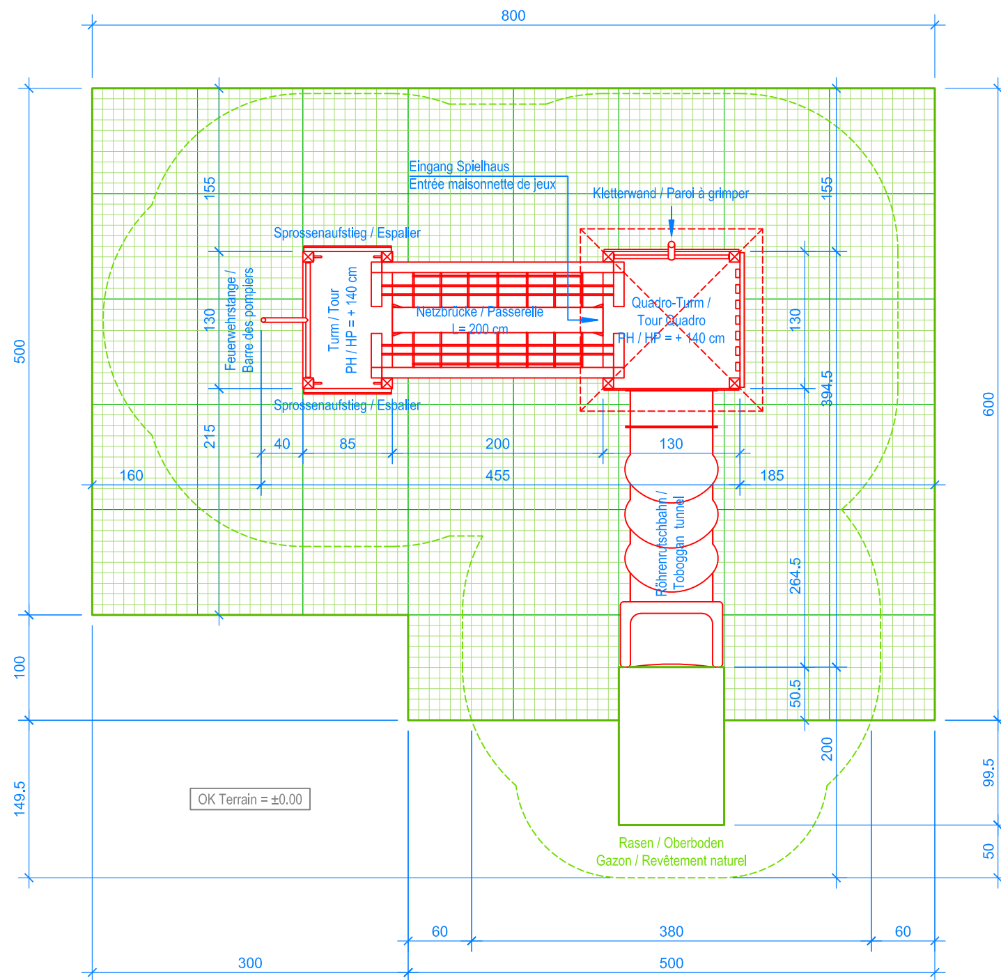
GRUNDRISS / PLAN 1:50
