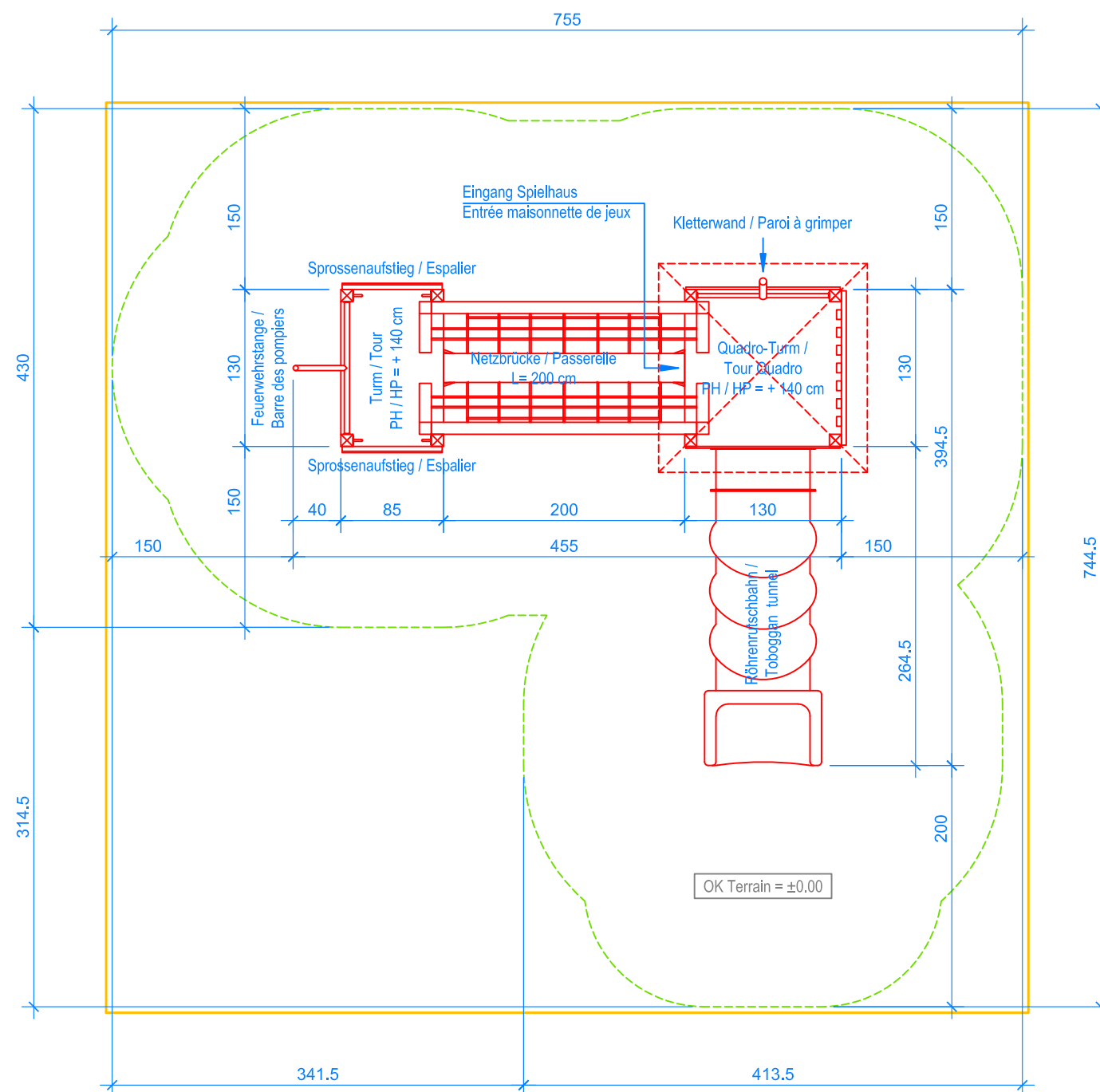
GRUNDRISS / PLAN 1:50
