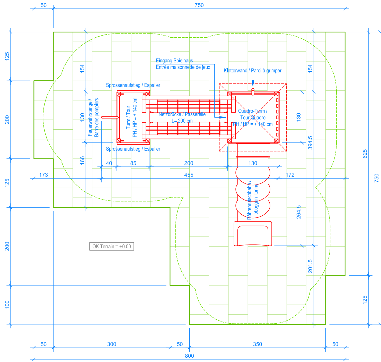
GRUNDRISS / PLAN 1:50
