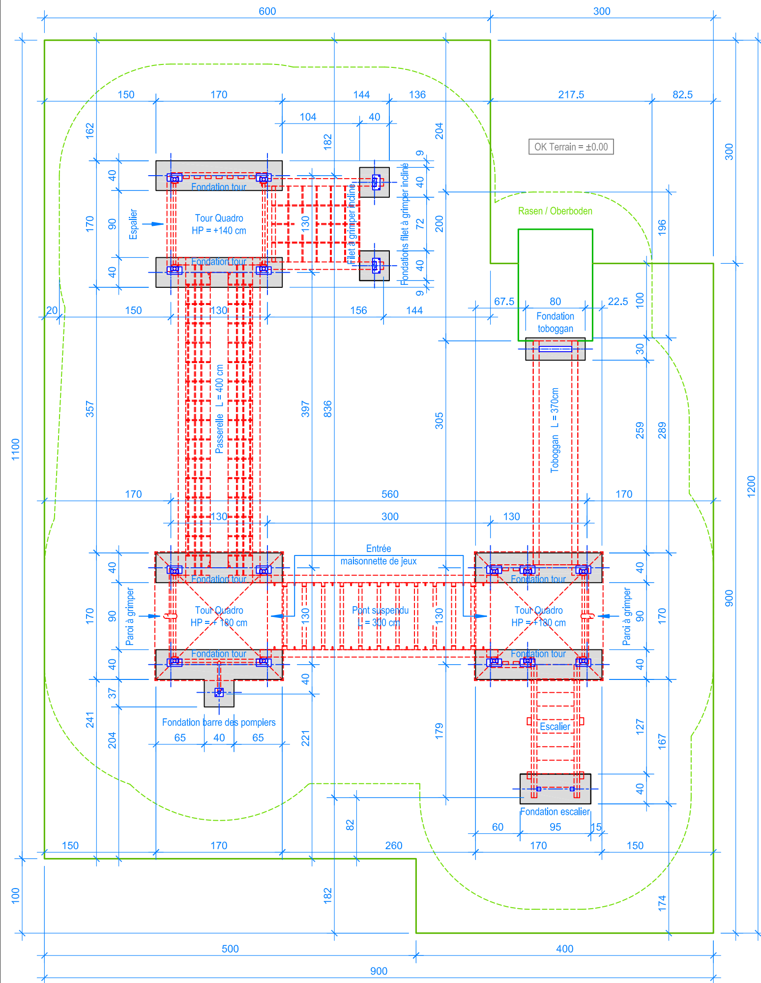
PLAN 1:50
