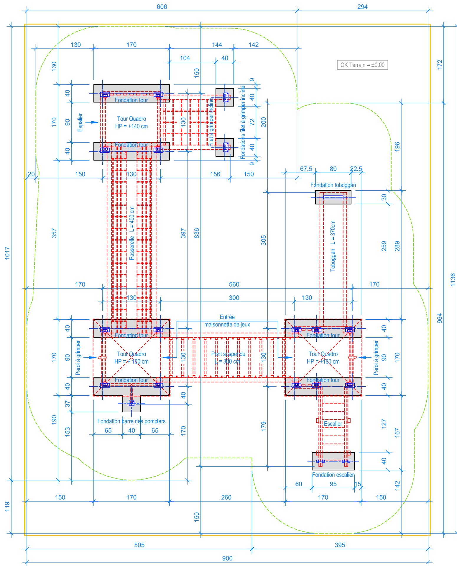
PLAN 1:50
