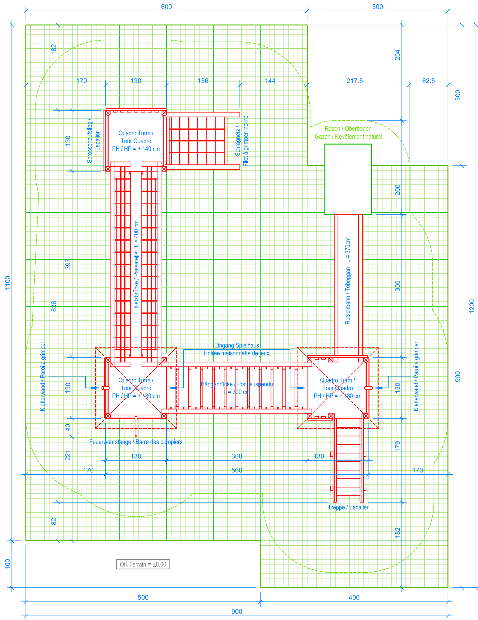
GRUNDRISS / PLAN 1:50
