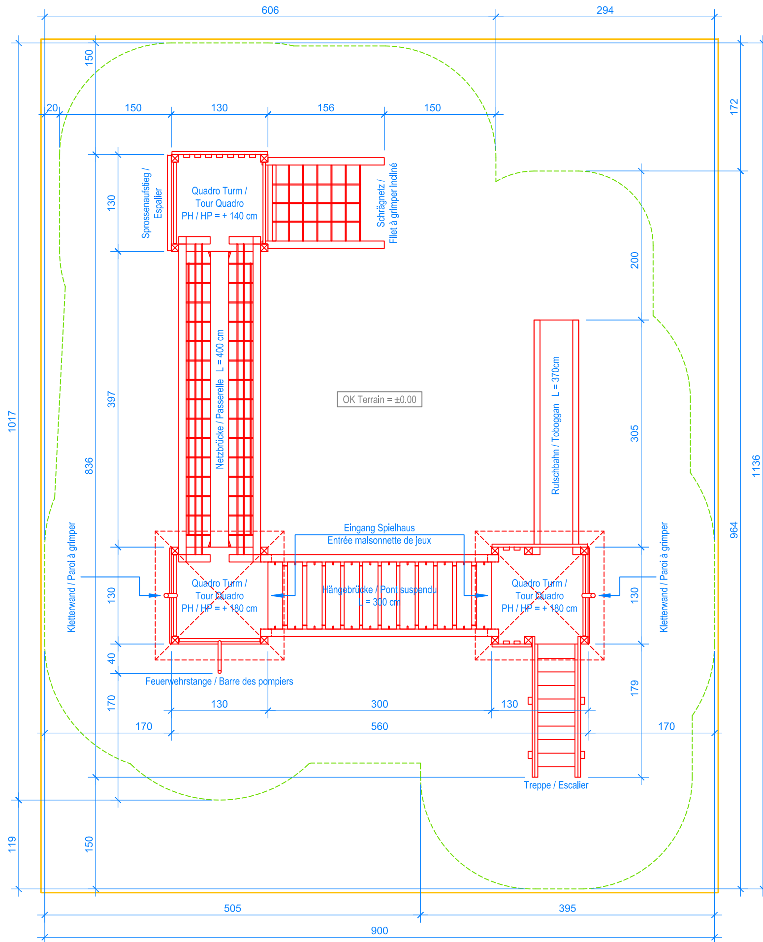
GRUNDRISS / PLAN 1:50
