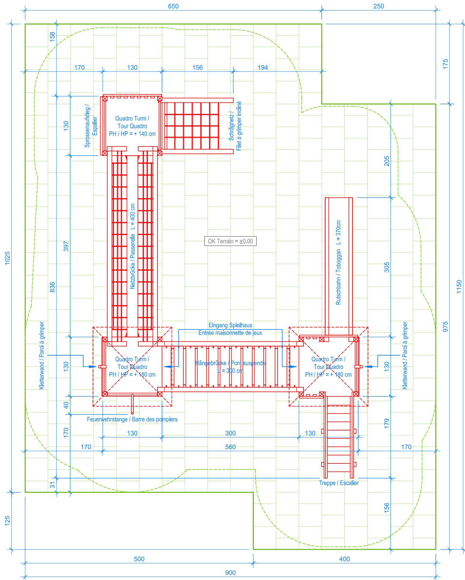
GRUNDRISS / PLAN 1:50
