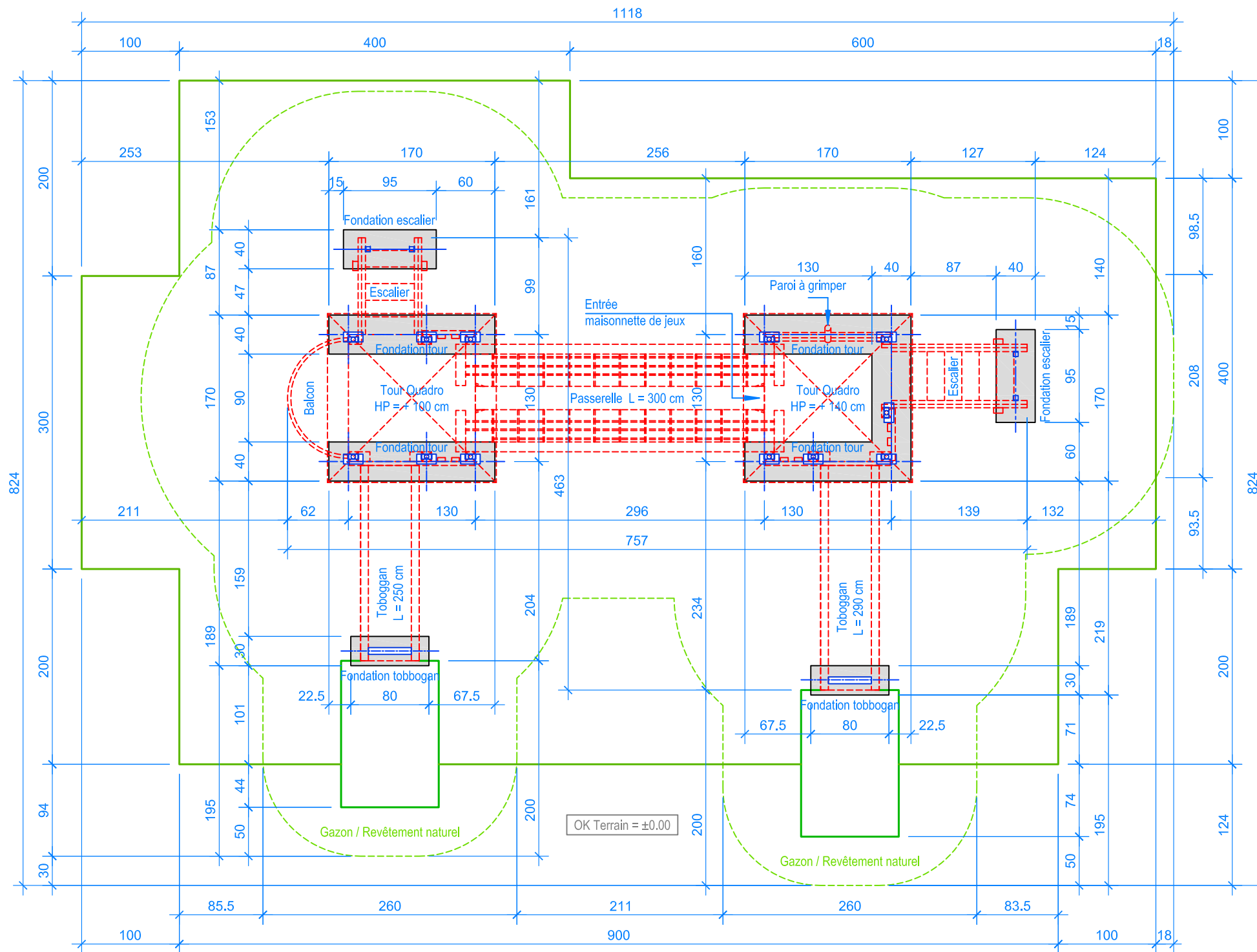
PLAN 1:50
