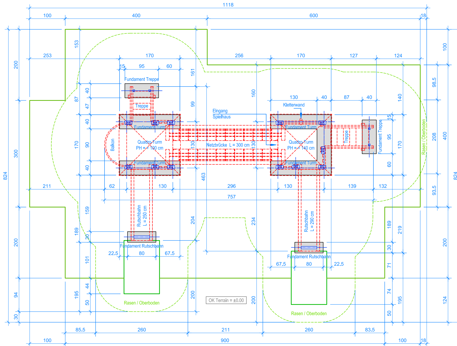
GRUNDRISS 1:50
