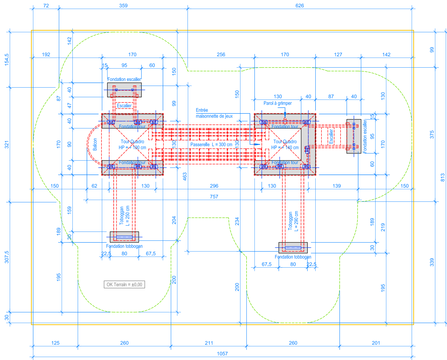
PLAN 1:50
