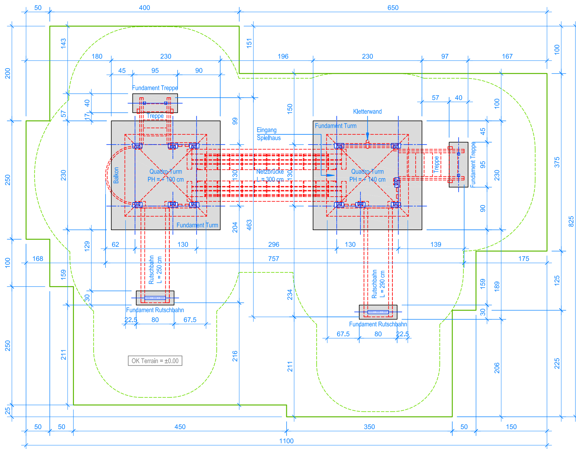
GRUNDRISS 1:50
