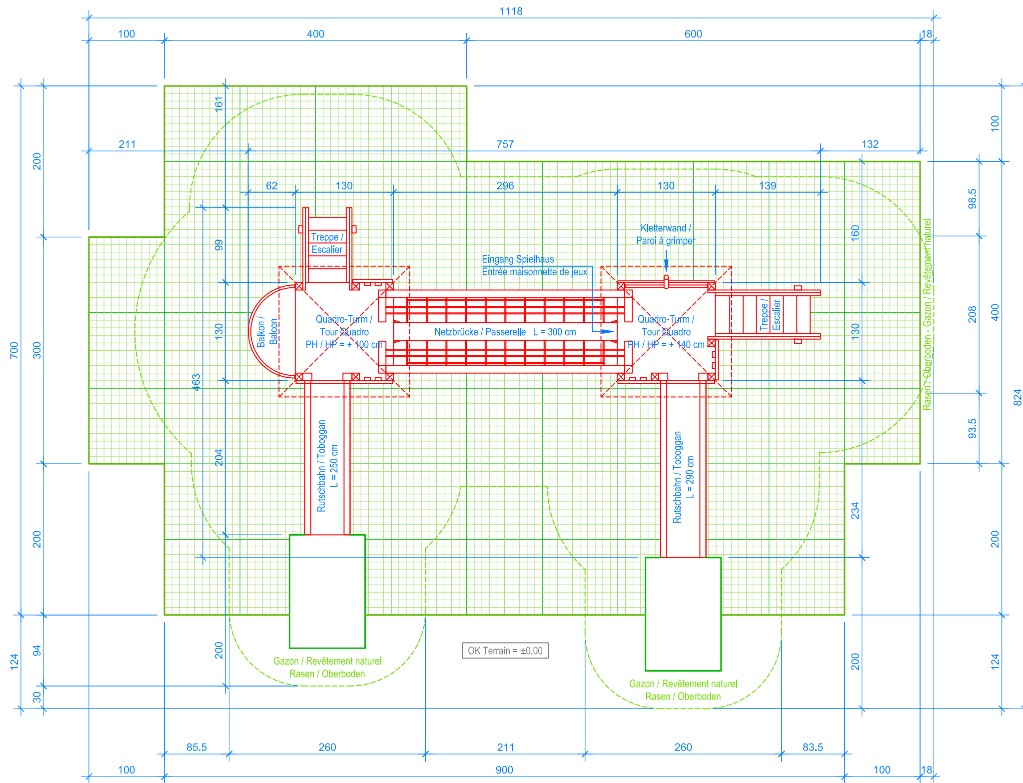
GRUNDRISS / PLAN 1:50
