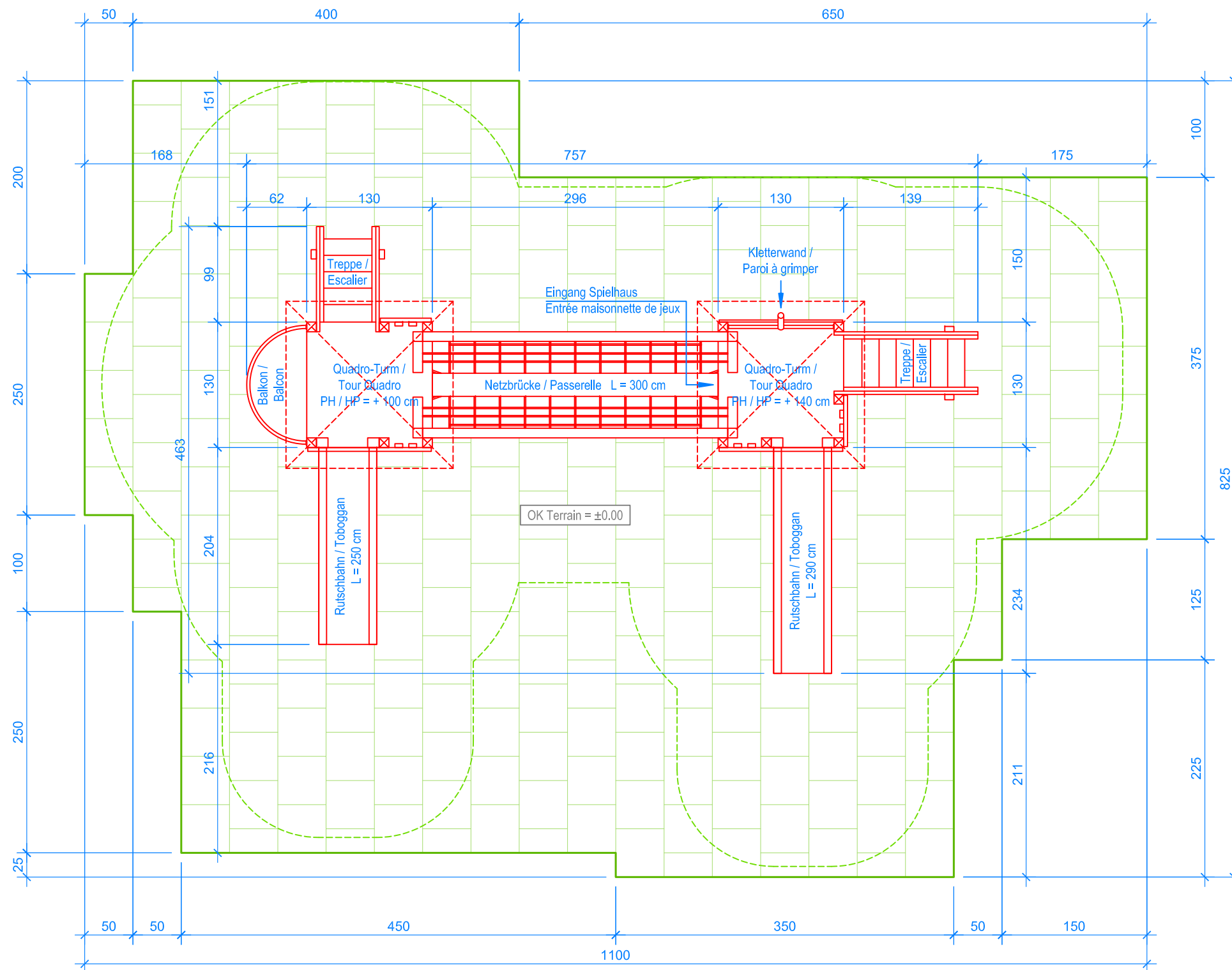
GRUNDRISS / PLAN 1:50
