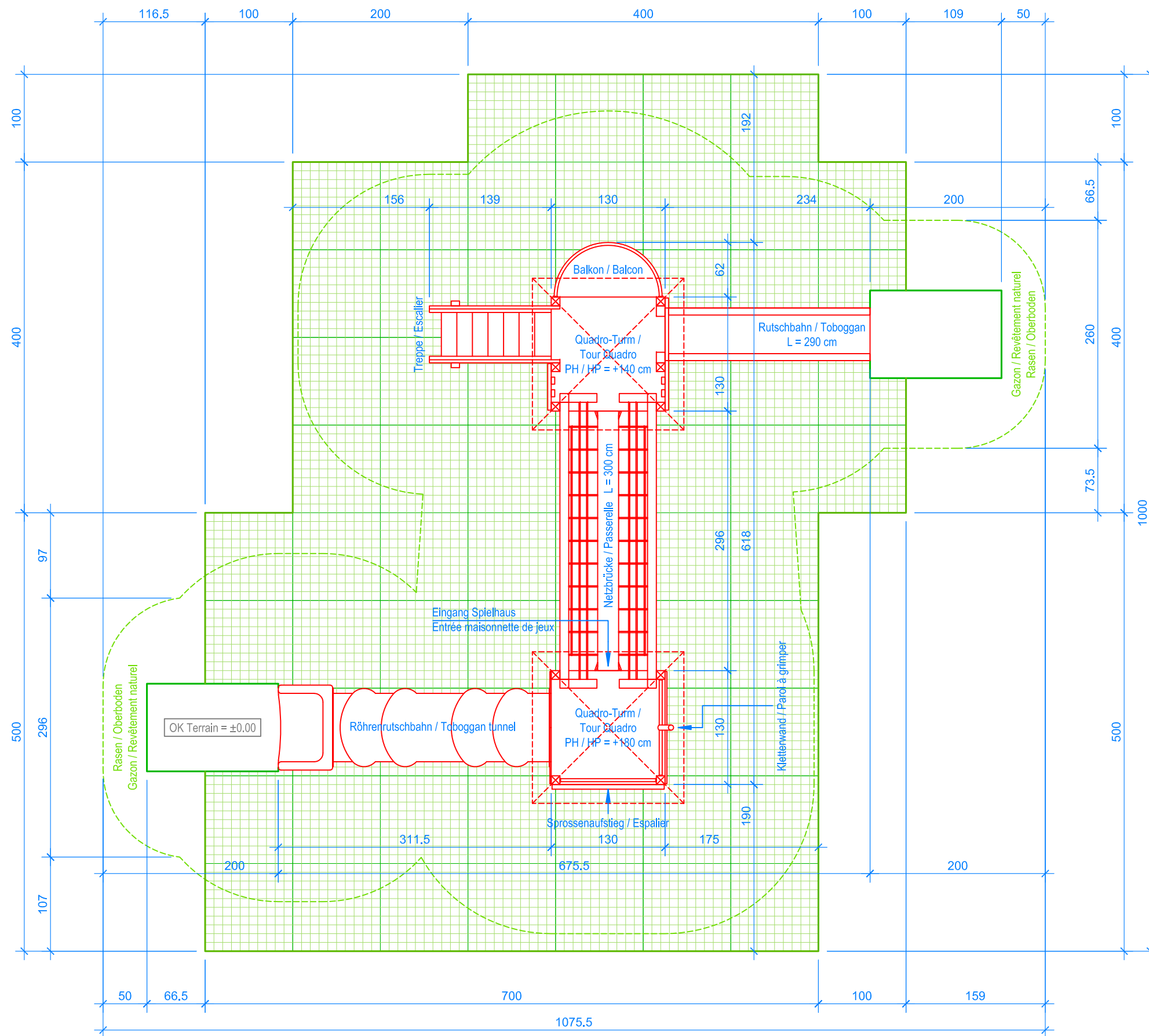
GRUNDRISS / PLAN 1:50
