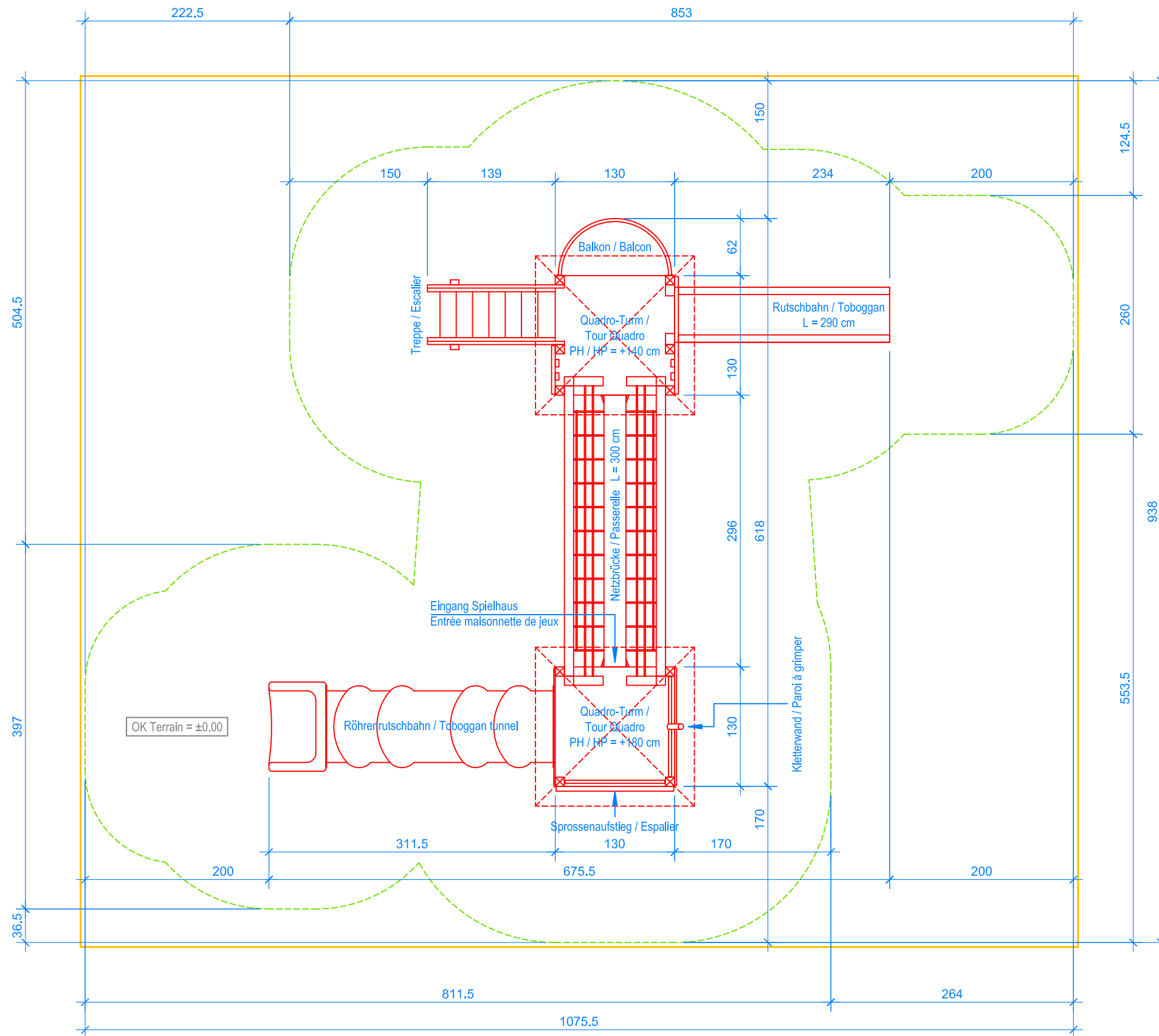
GRUNDRISS / PLAN 1:50
