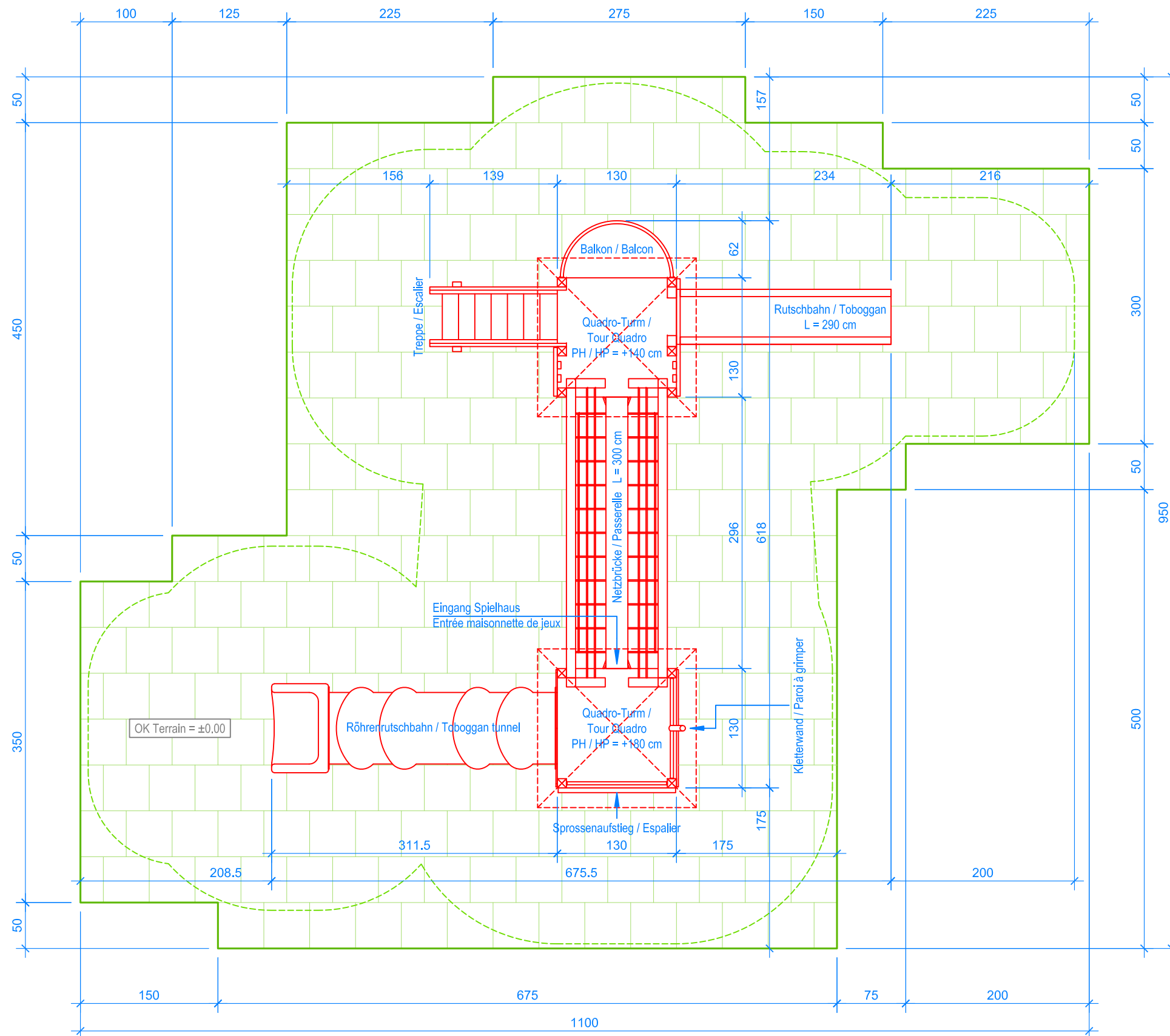
GRUNDRISS / PLAN 1:50
