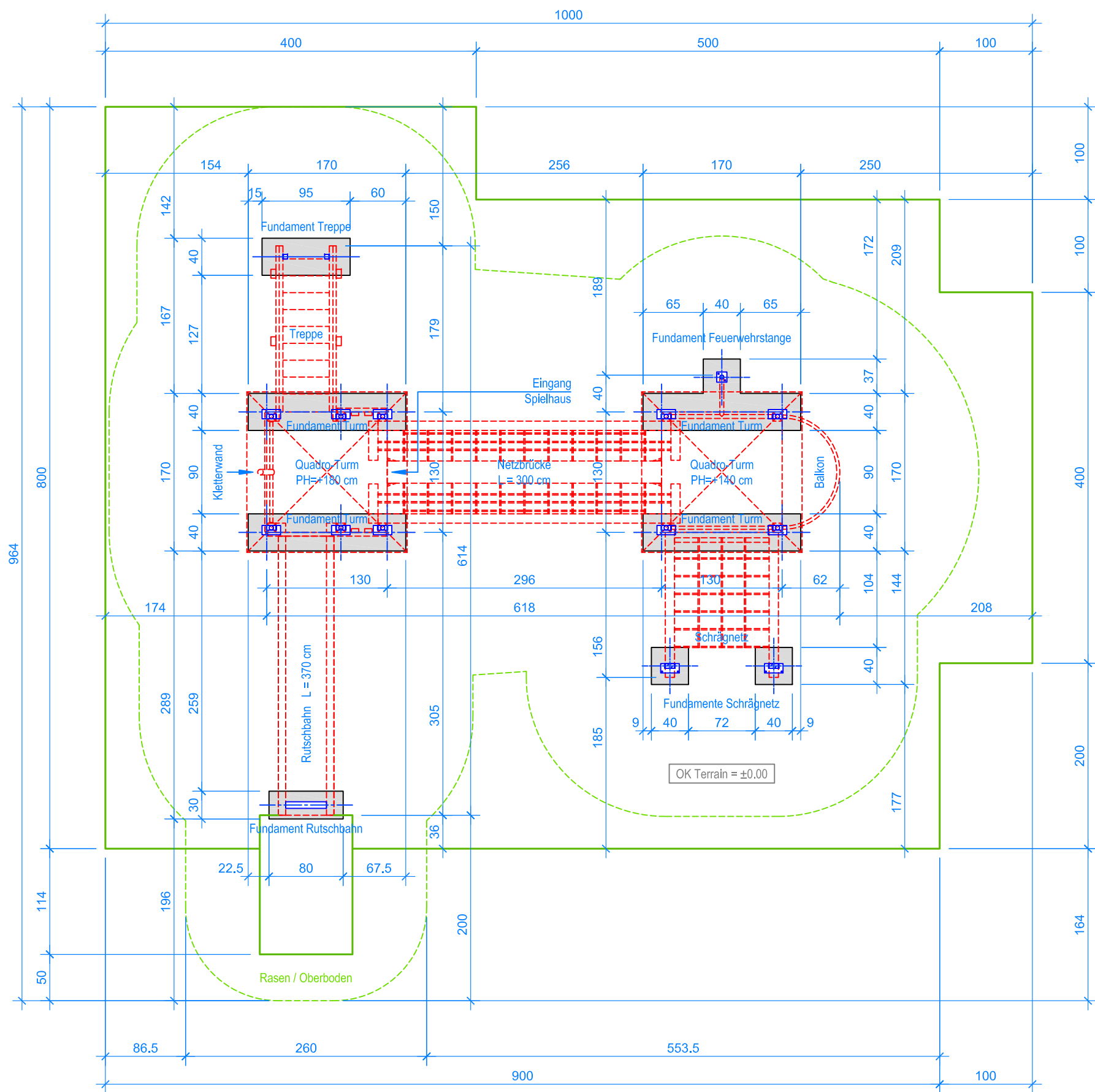
GRUNDRISS 1:50
