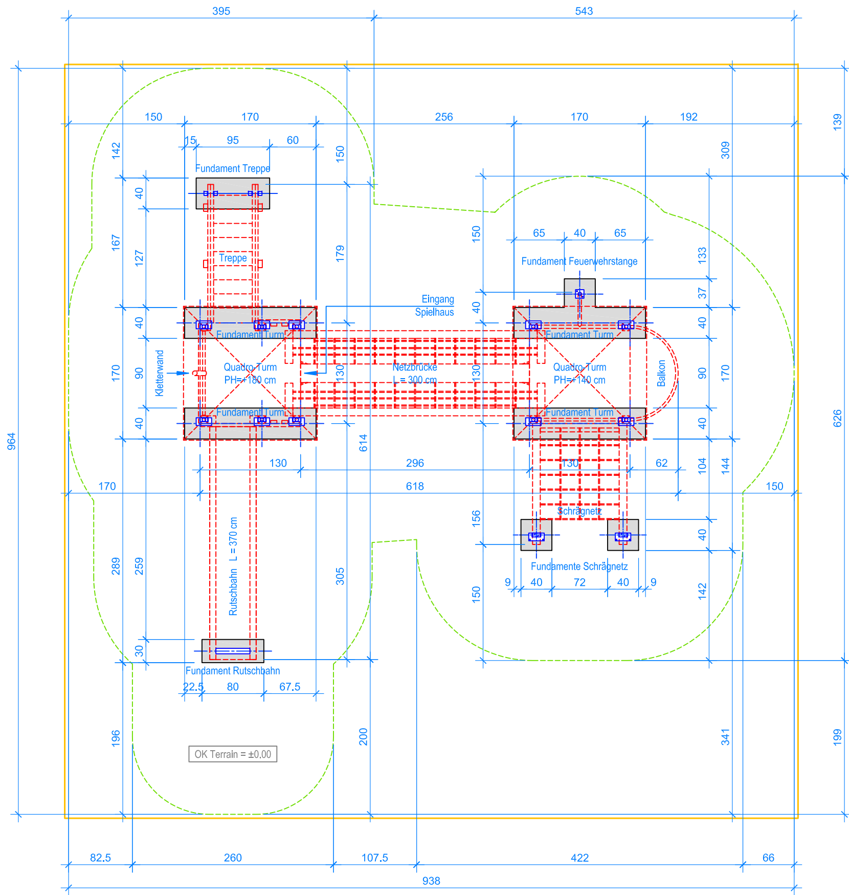
GRUNDRISS 1:50
