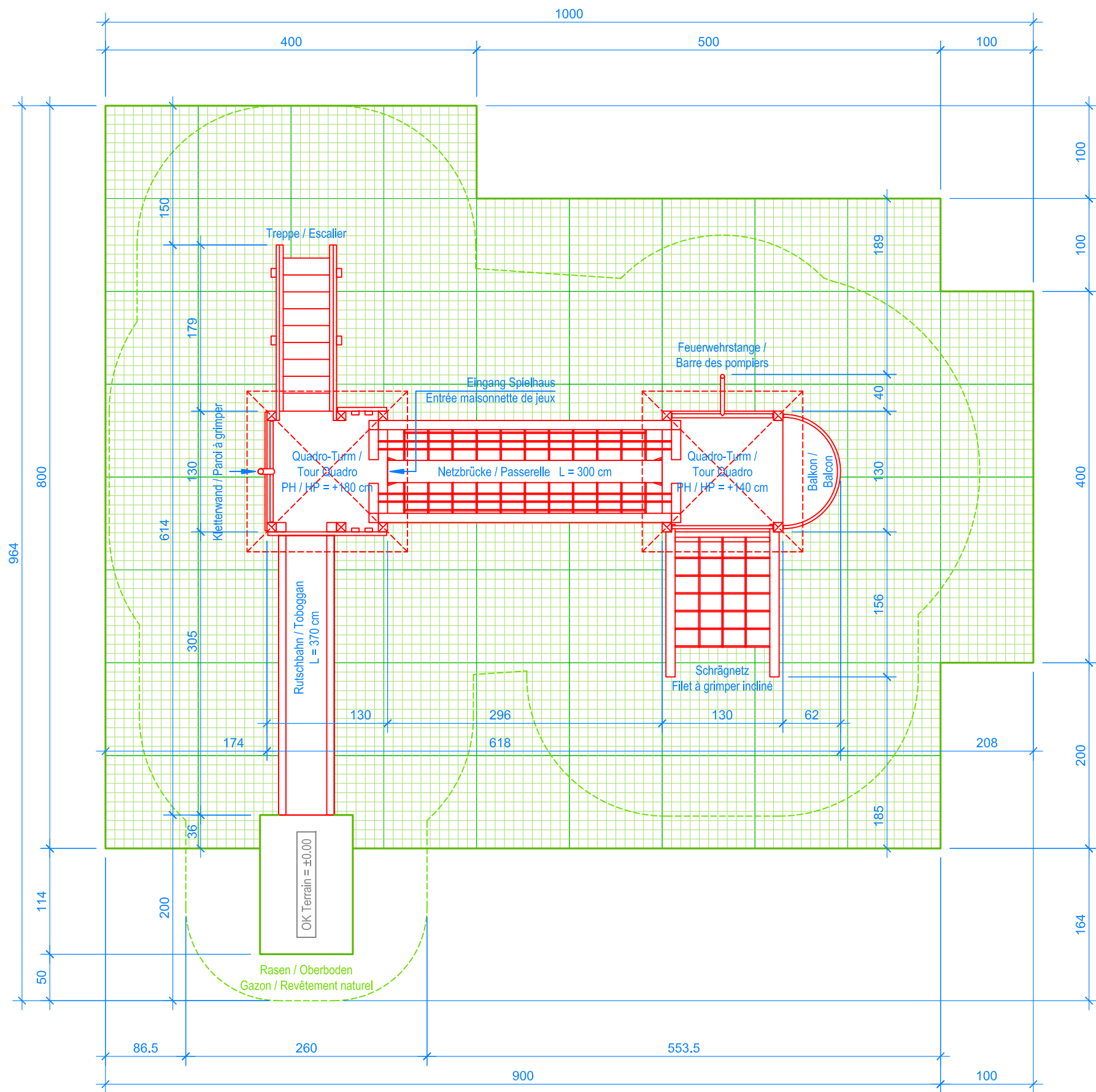
GRUNDRISS / PLAN 1:50
