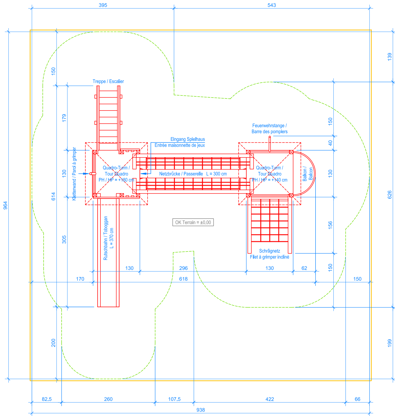
GRUNDRISS / PLAN 1:50
