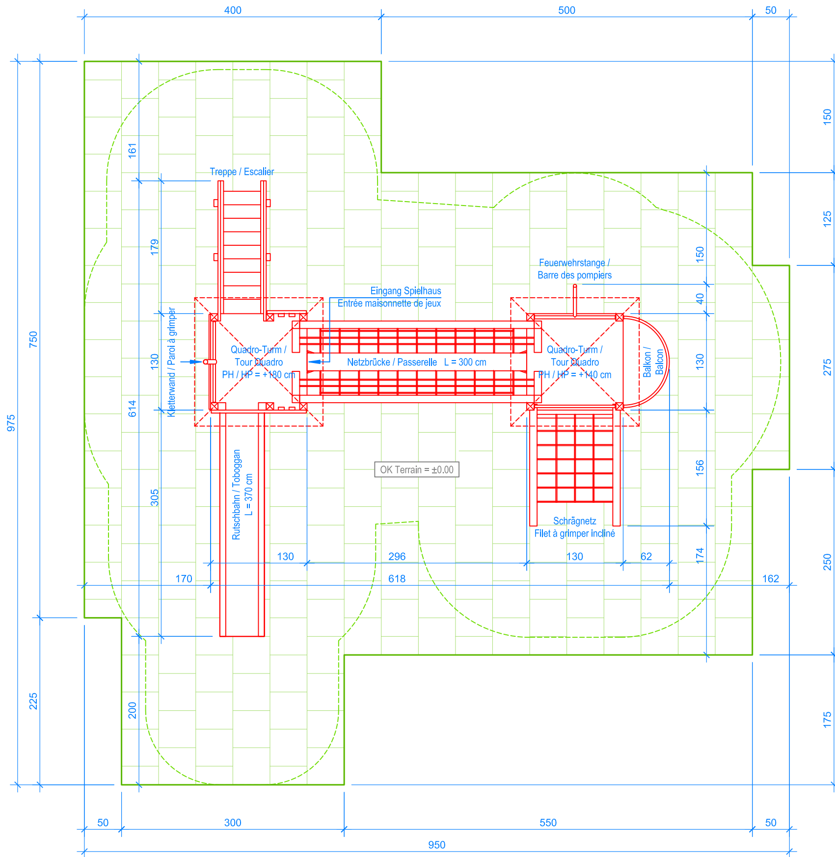
GRUNDRISS / PLAN 1:50
