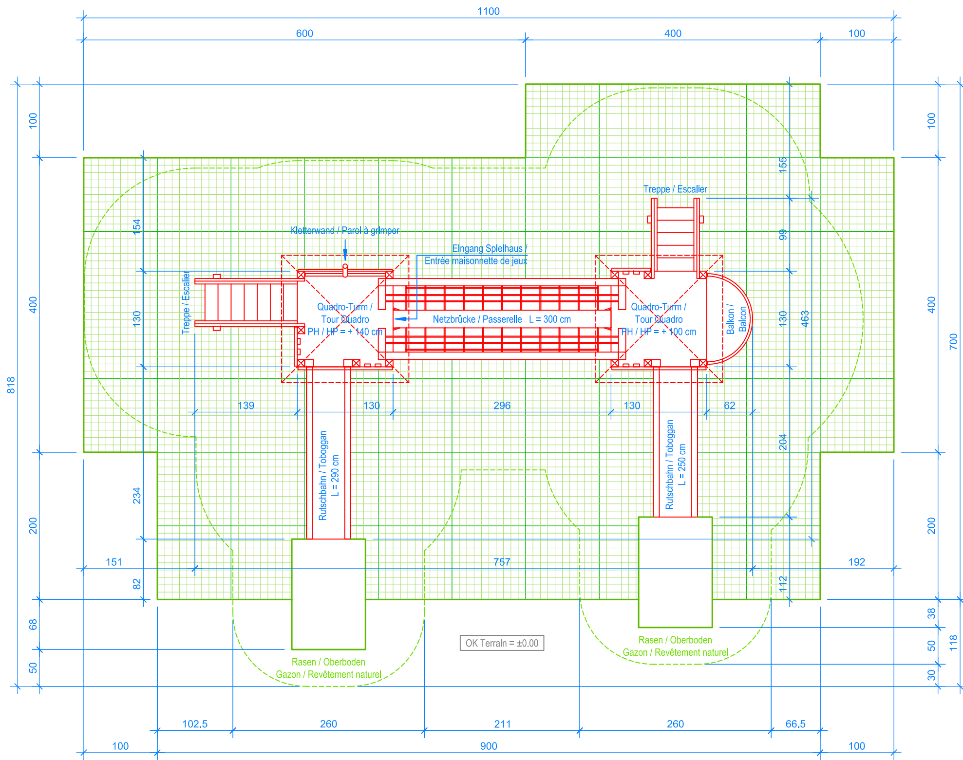
GRUNDRISS / PLAN 1:50
