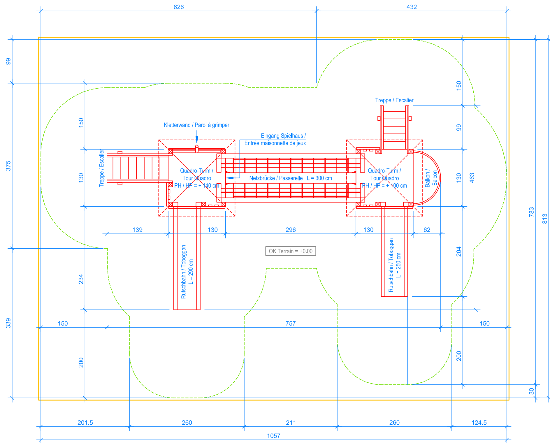
GRUNDRISS / PLAN 1:50
