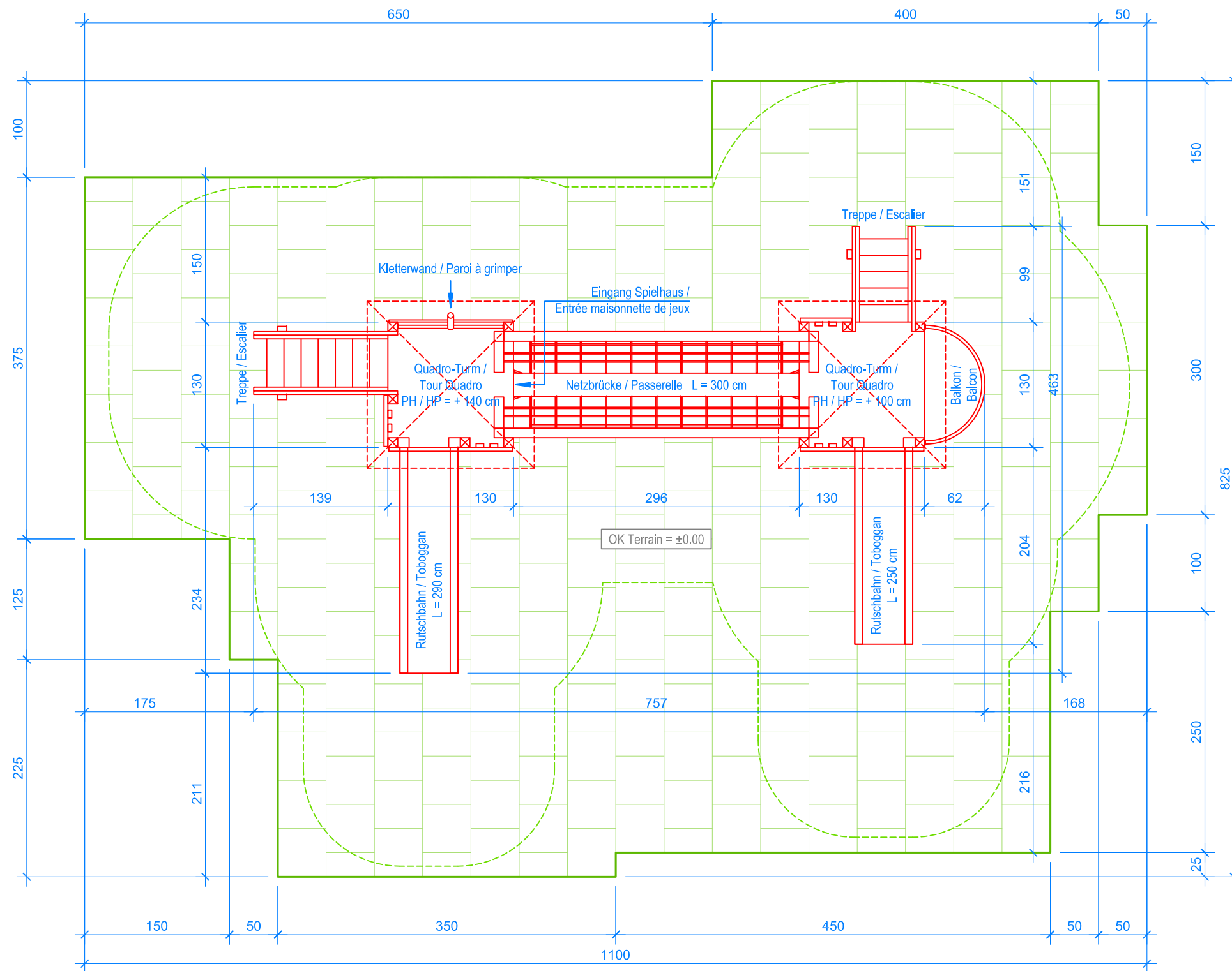
GRUNDRISS / PLAN 1:50
