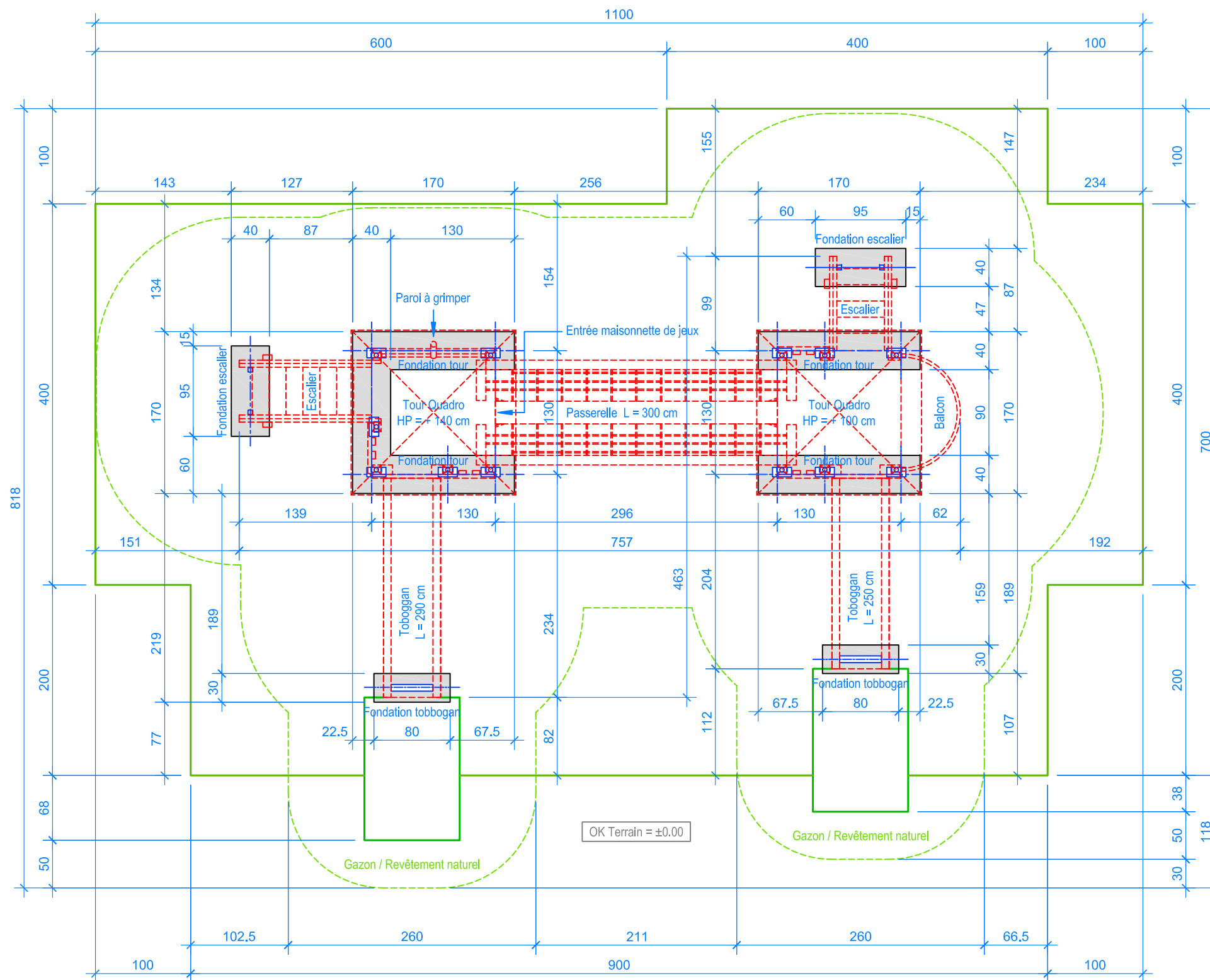
PLAN 1:50
