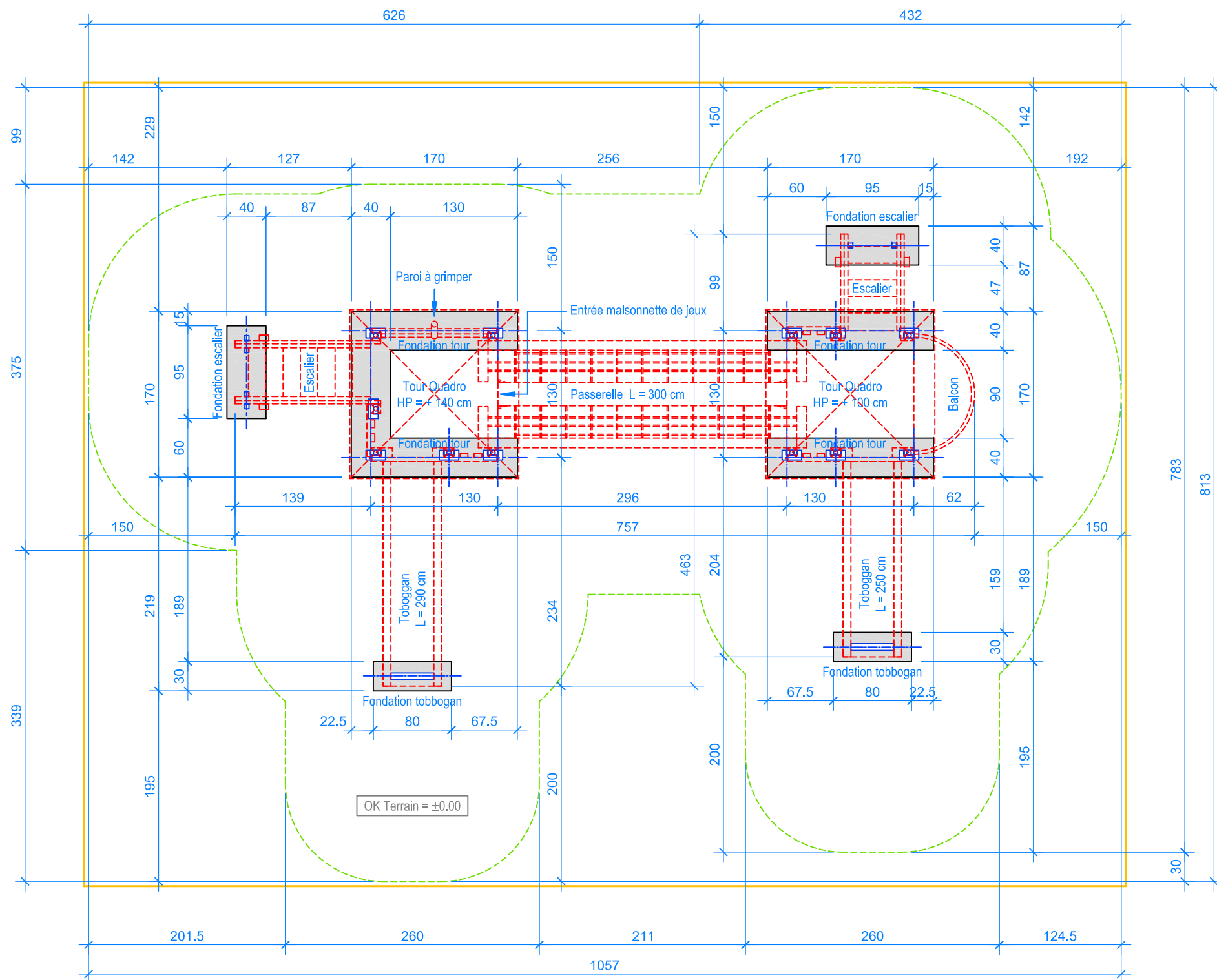
PLAN 1:50
