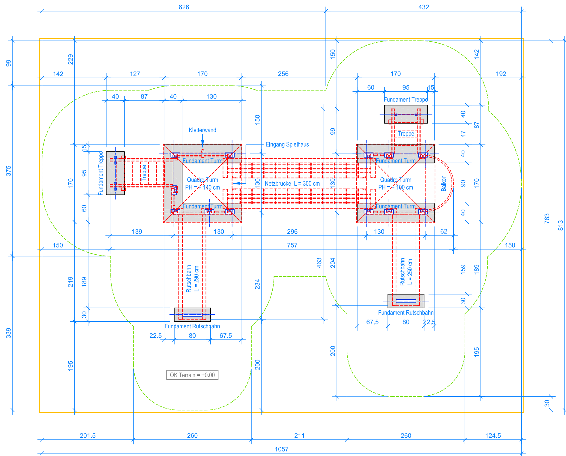
GRUNDRISS 1:50
