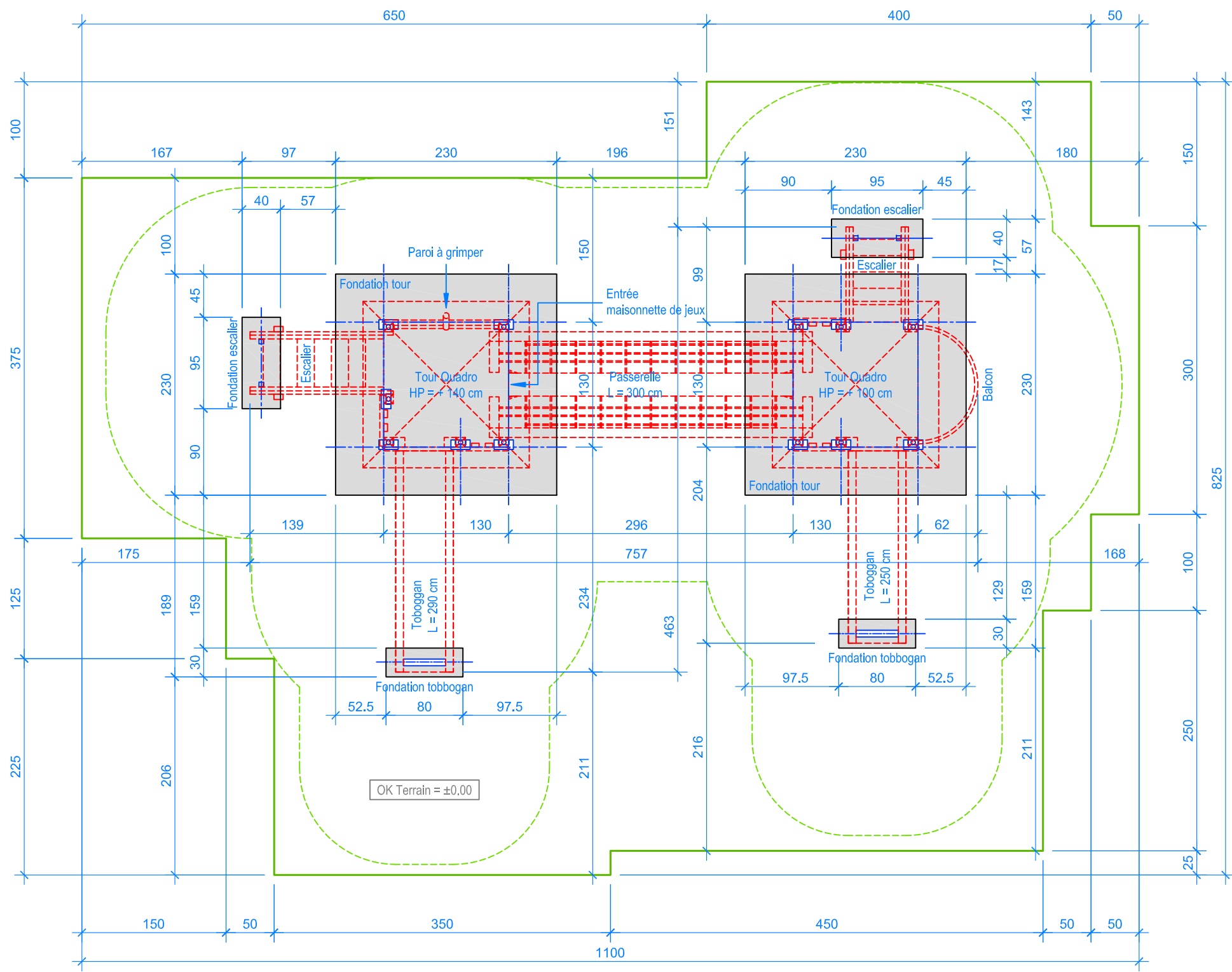
PLAN 1:50
