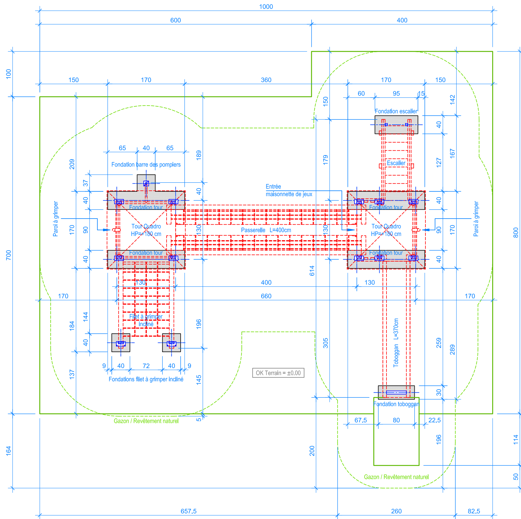
PLAN 1:50
