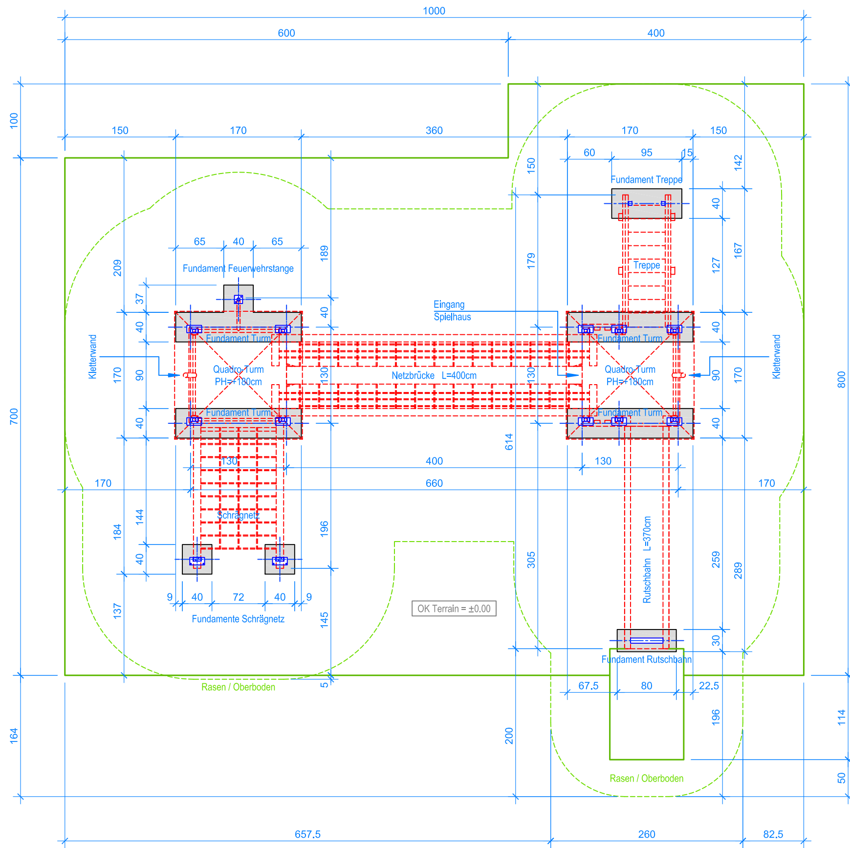
GRUNDRISS 1:50
