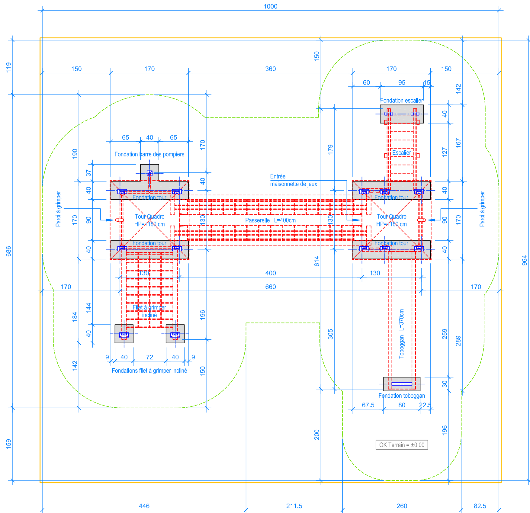
PLAN 1:50
